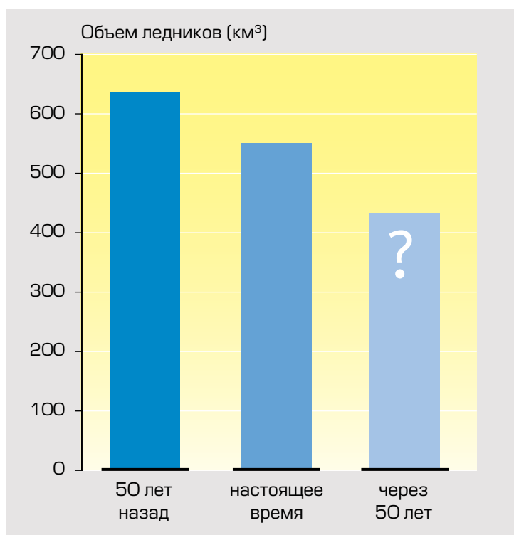
Рисунок 4.2. Изменение объема ледников Таджикистана
